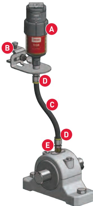
Ejemplo de montaje de lubricación de rodamientos
